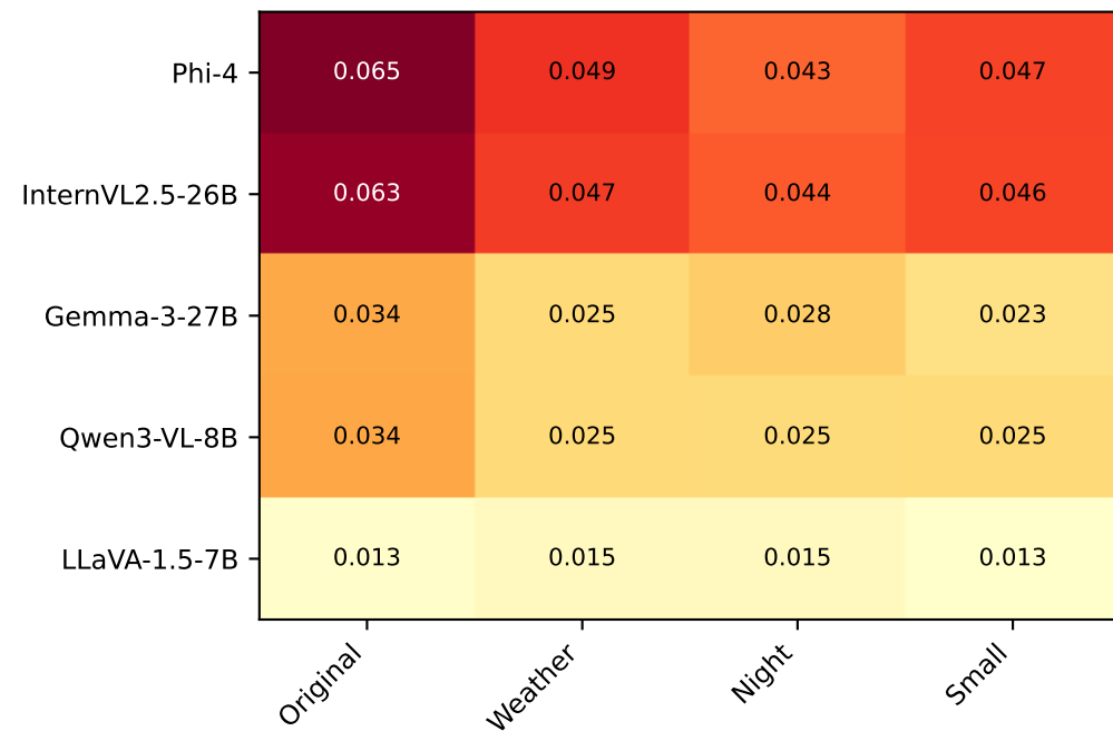
BLEU
