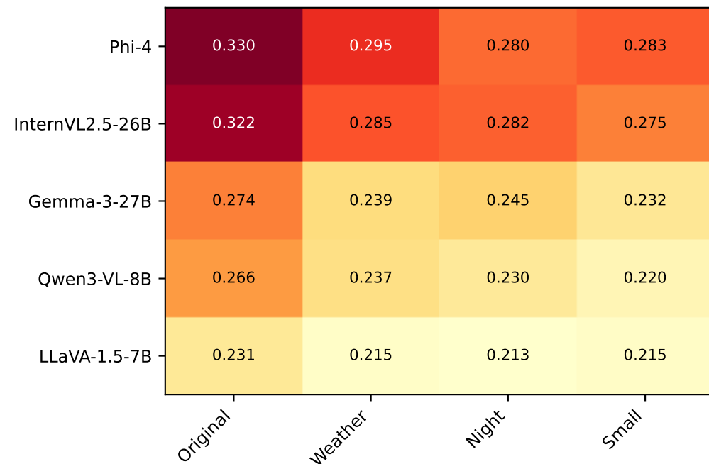
BERT-F1
