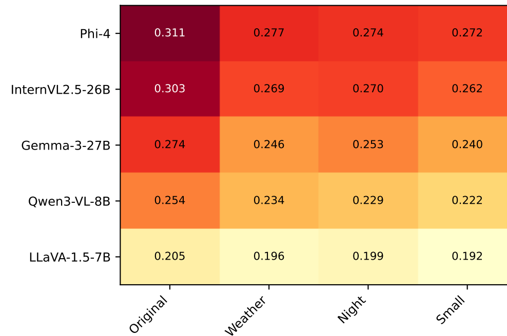
ROUGE-L
