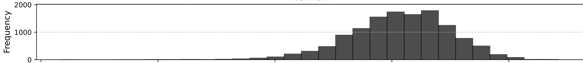
GPT
