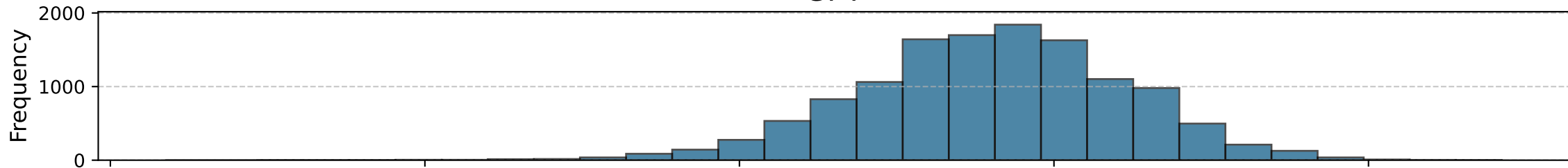
LLaMA
