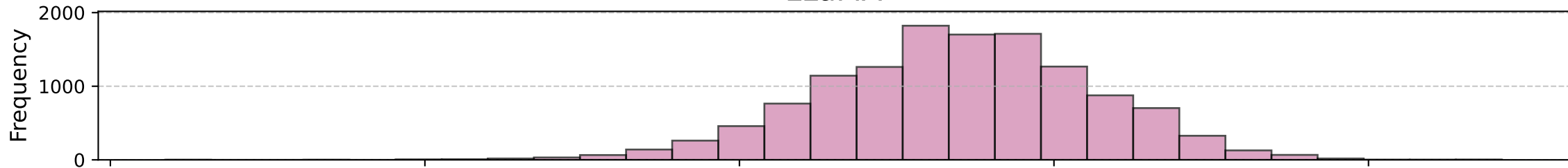
Pegasus
