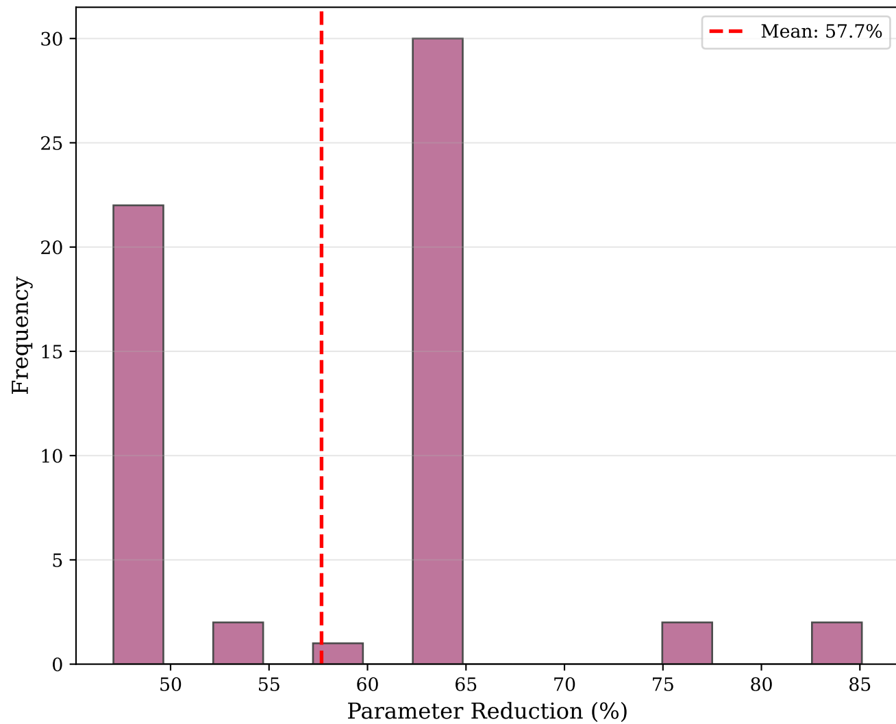
Parameter Reduction Distribution
