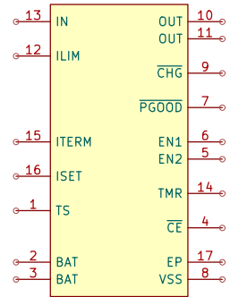
U6 BQ24074RGTR
