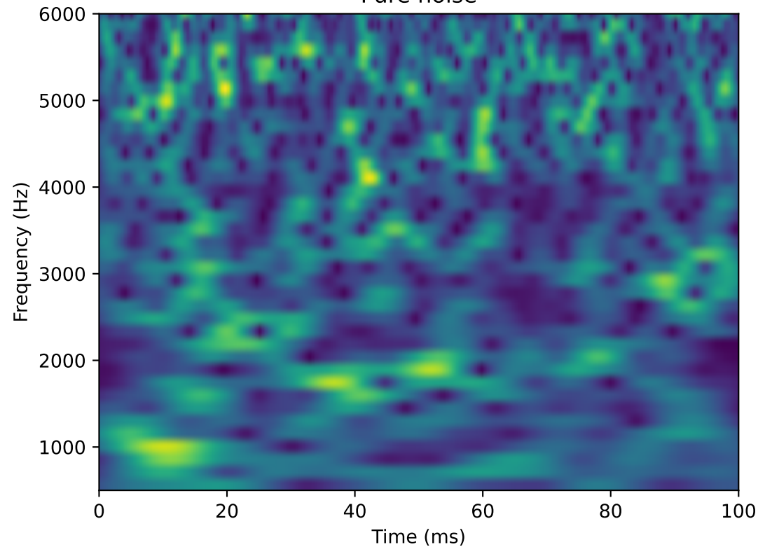
Pure noise
