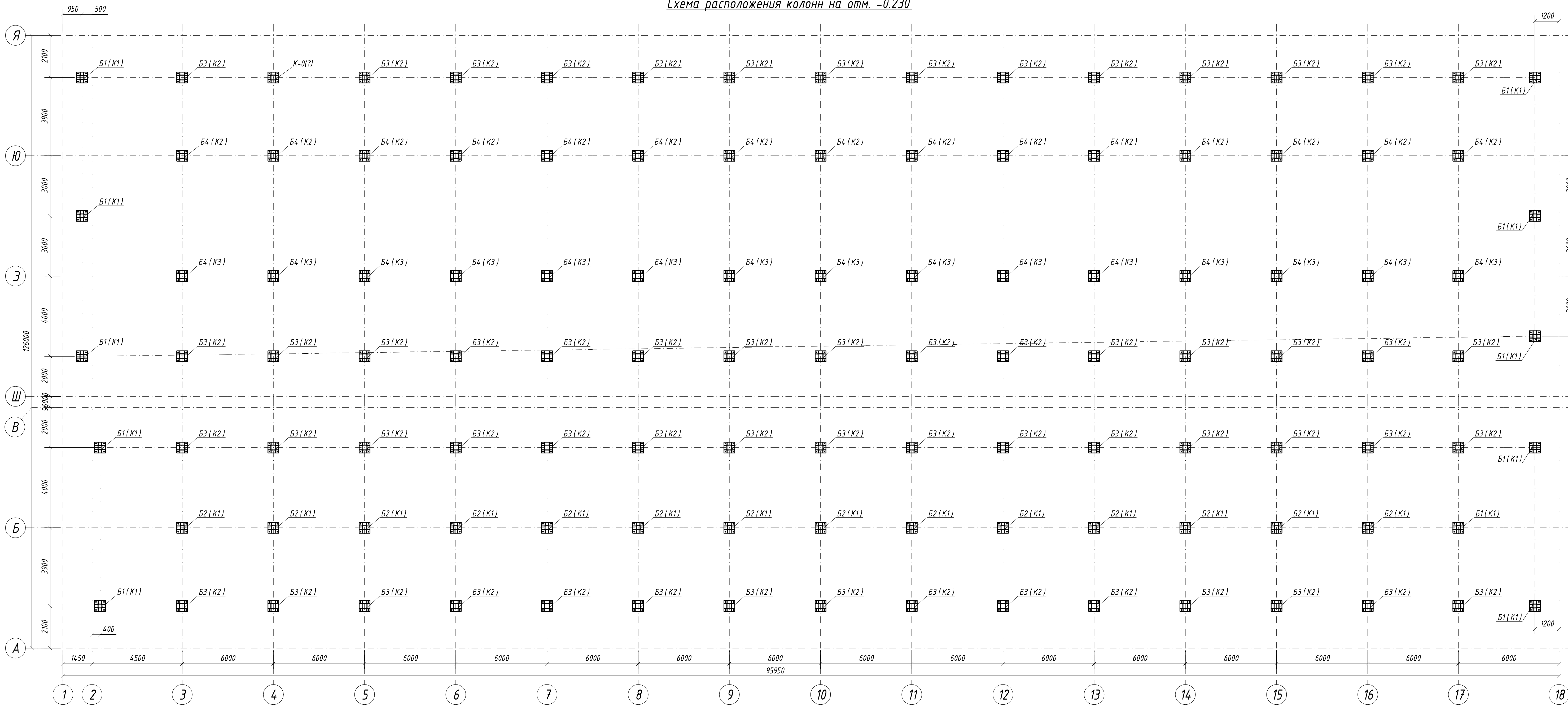
Схема расположения колонн на отм. -0.230
