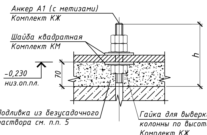
Деталь "А"
