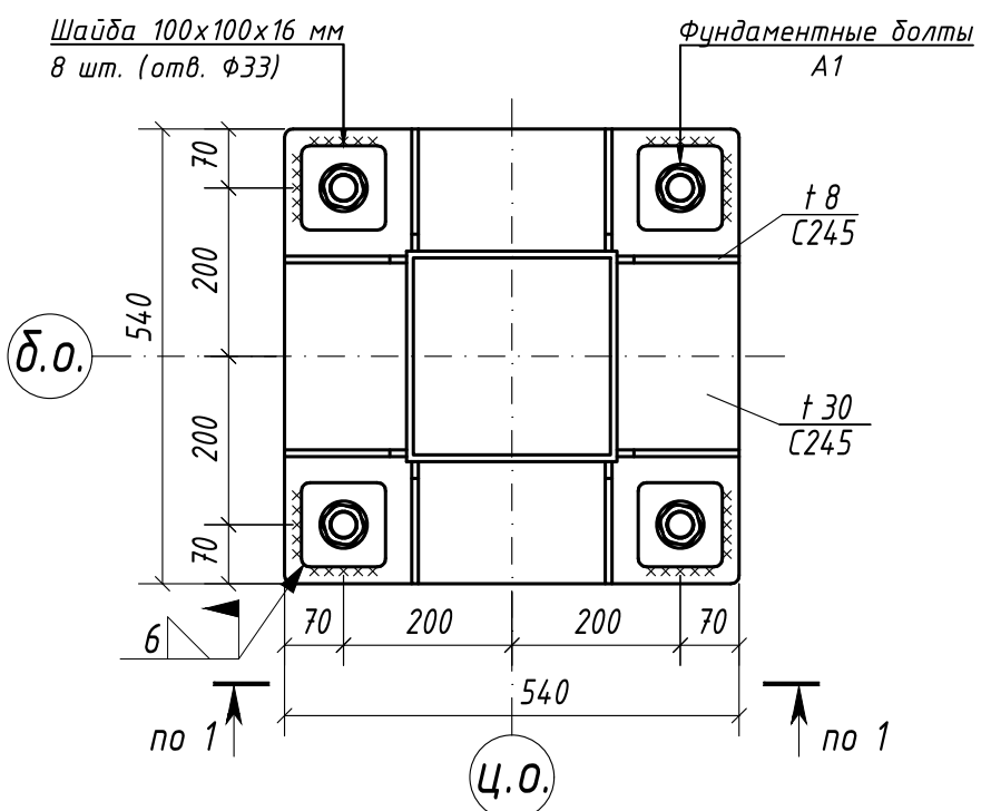
База колонн Б3, Б4
