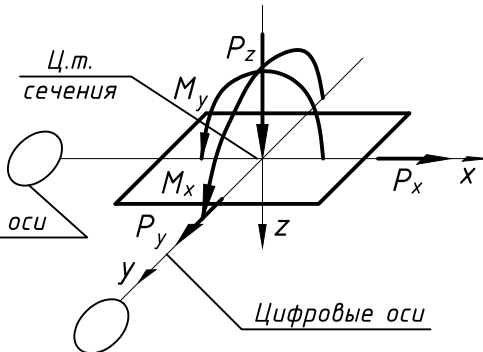
Схема нагрузок и правило знаков
