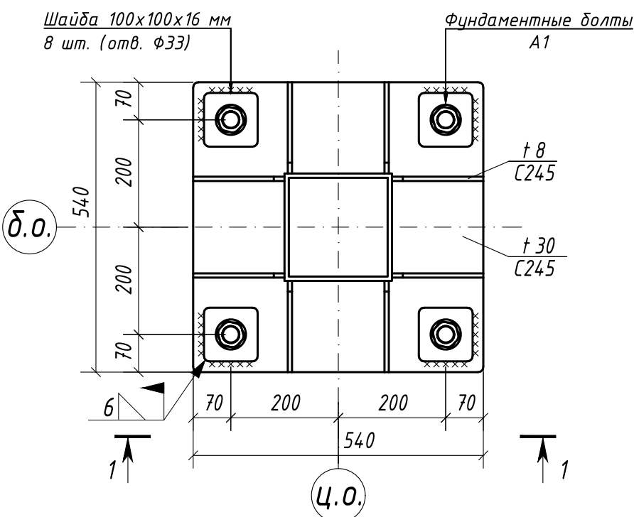
База колонн Б1, Б2
