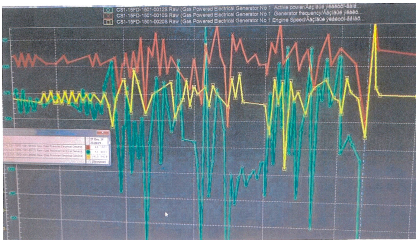
Приложение №1/ Attachment #1. Тренд рабочих параметров ГПЭС №1 / Trend of operating parameters of the GPPG #1.
