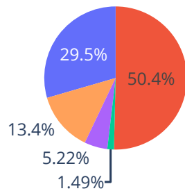
lldb (CLI)
