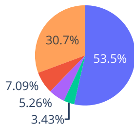
lldb (CLI)
