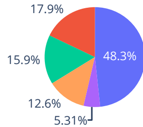
gdb (CLI)
