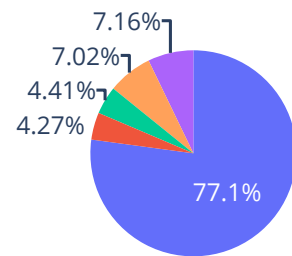
gdb (CLI)
