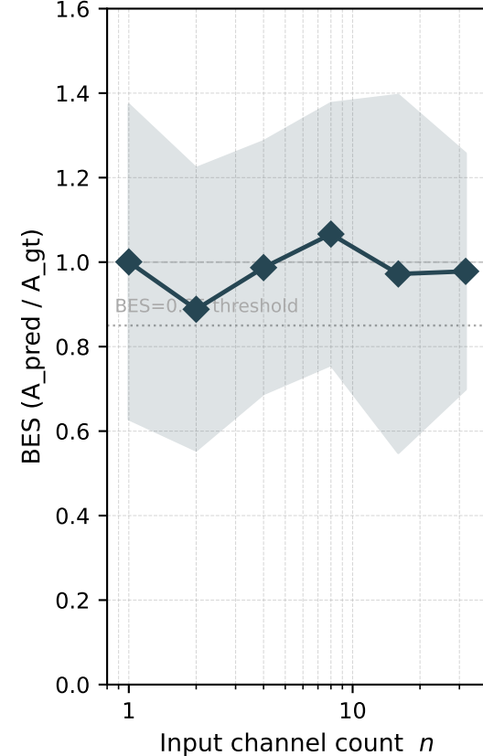
BES Scaling (ZUNA)
