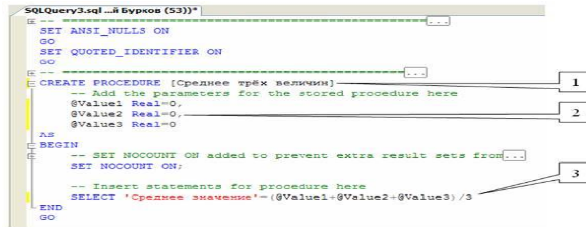
3 сурет - Процедуралардың кодтарын теретін терезе
