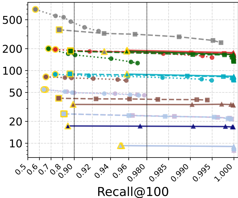
Rerank QPS
