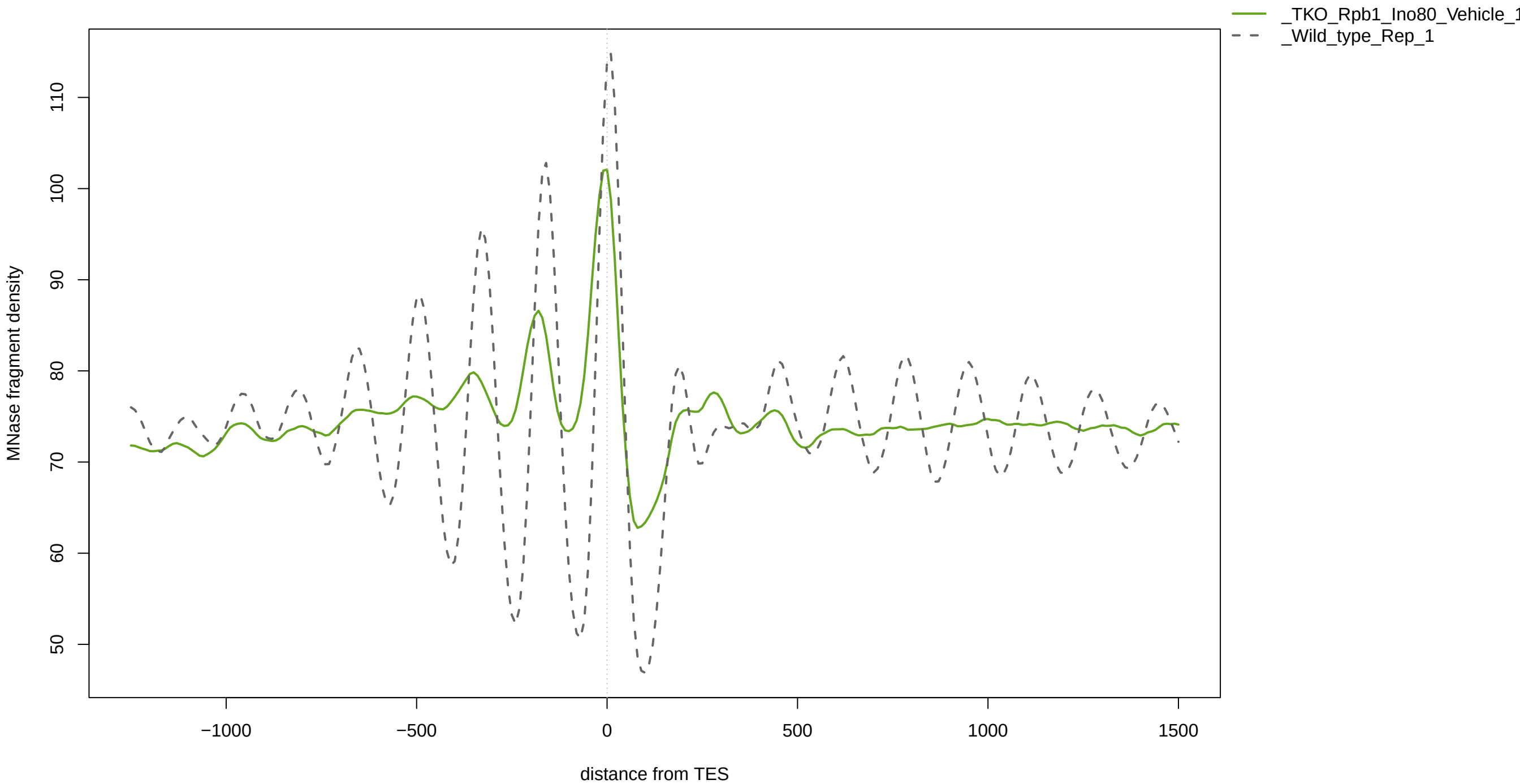
_TKO_Rpb1_Ino80_Vehicle_120_min_Rep_1 vs _Wild_type_Rep_1
