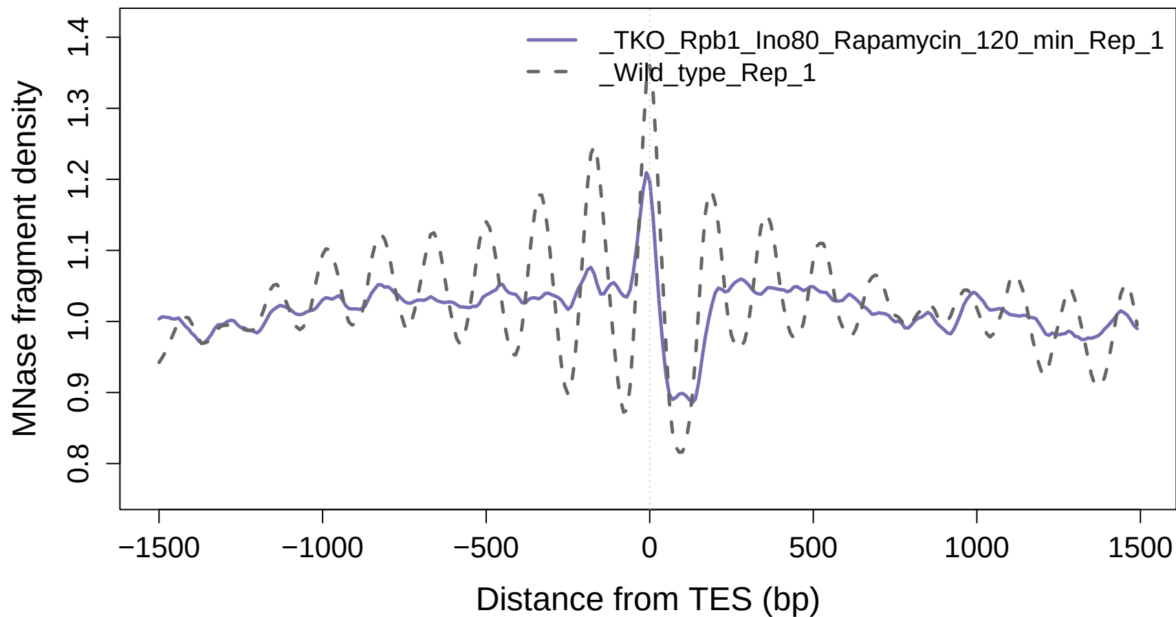
_TKO_Rpb1_Ino80_Rapamycin_120_min_Rep_1 vs _Wild_type_Rep_1 (conv
