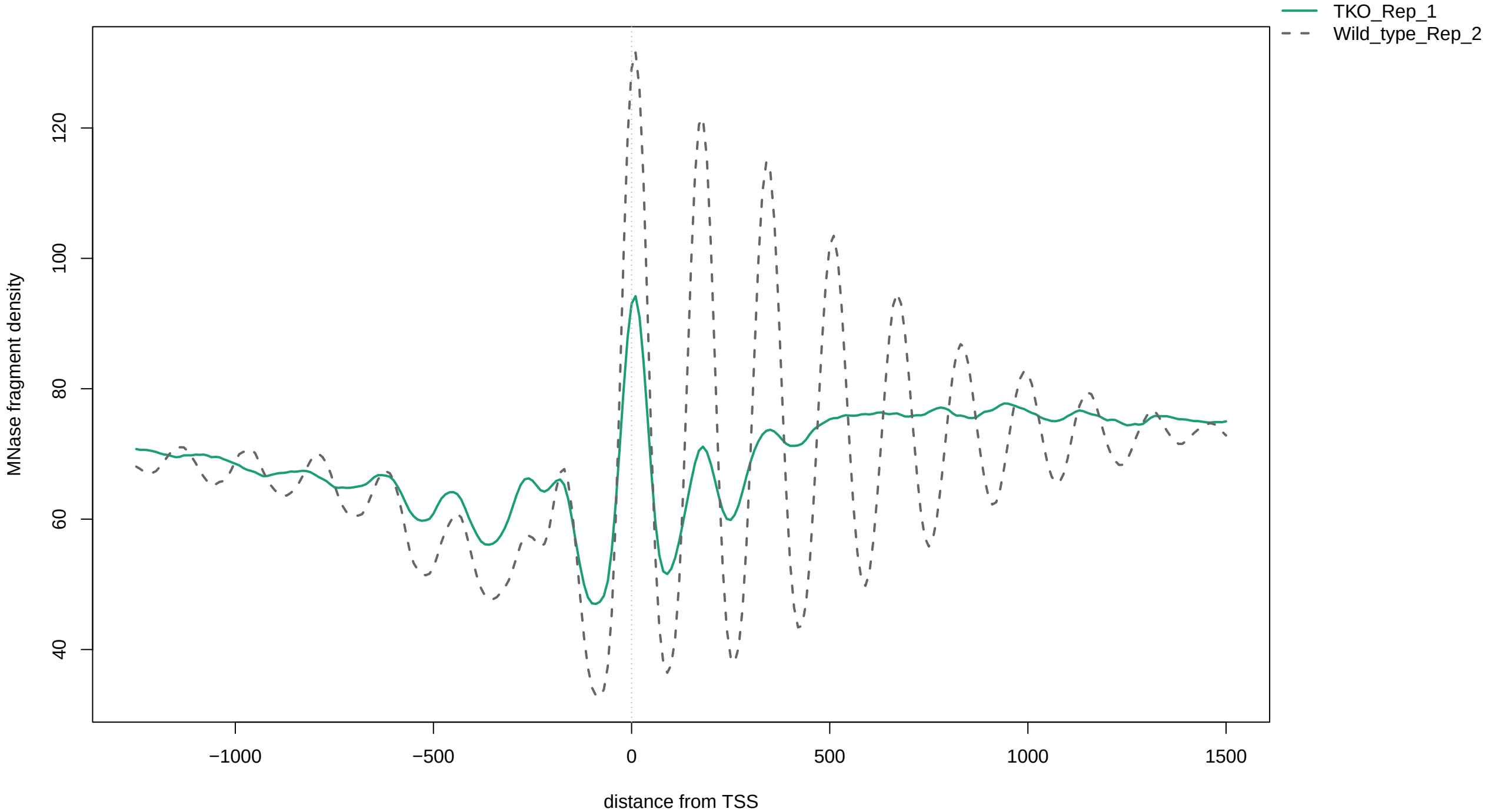
TKO_Rep_1 vs Wild_type_Rep_2
