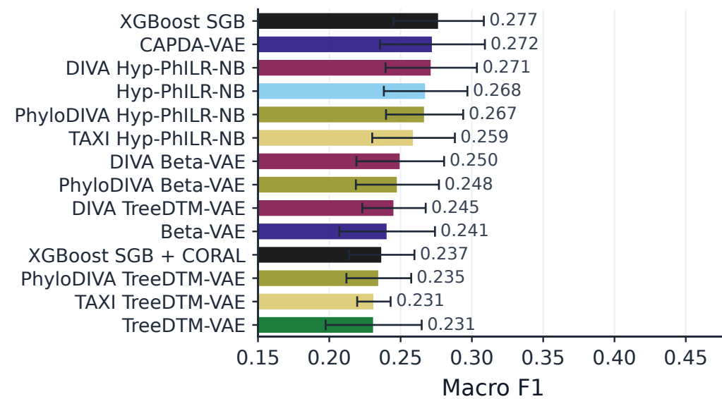
Strict LOSO macro F1
