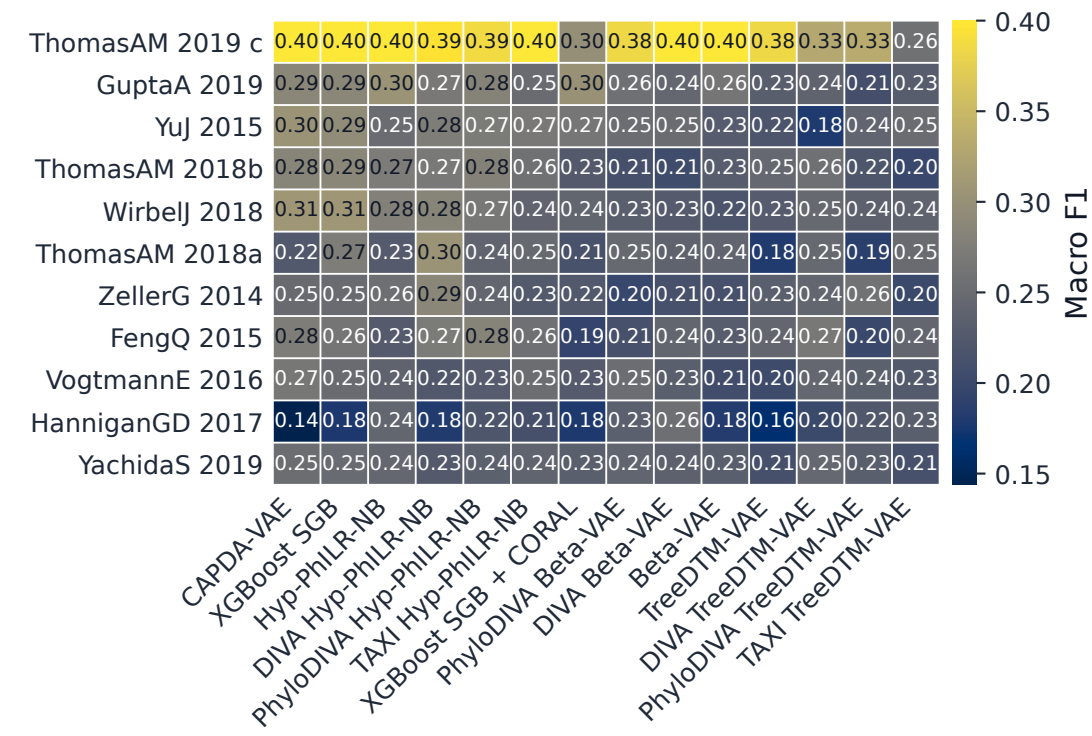
Macro F1 by held-out study
