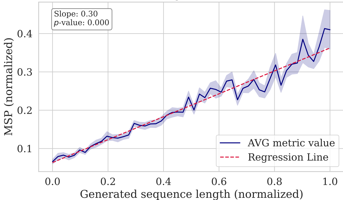
MSP vs. Length (WMT14 Cs-En)
