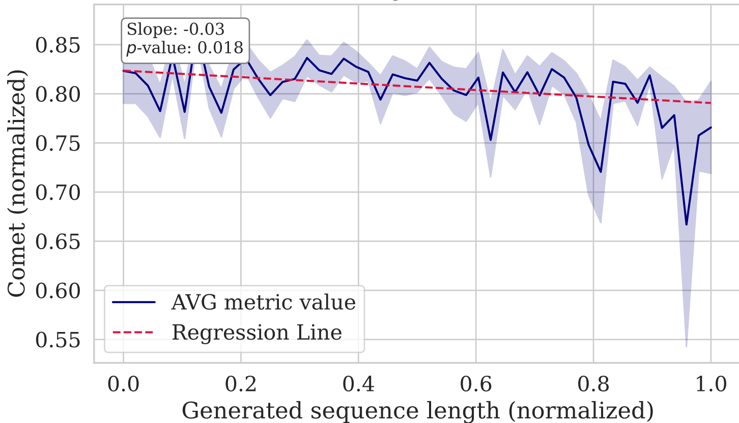
Comet vs. Length (WMT14 Cs-En)
