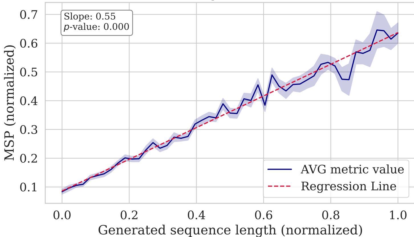
MSP vs. Length (WMT14 Cs-En)
