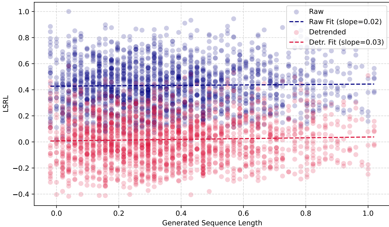
LSRL vs. Length (WMT14 Cs-En)
