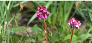
Bergénie Bergenia cordifolia
