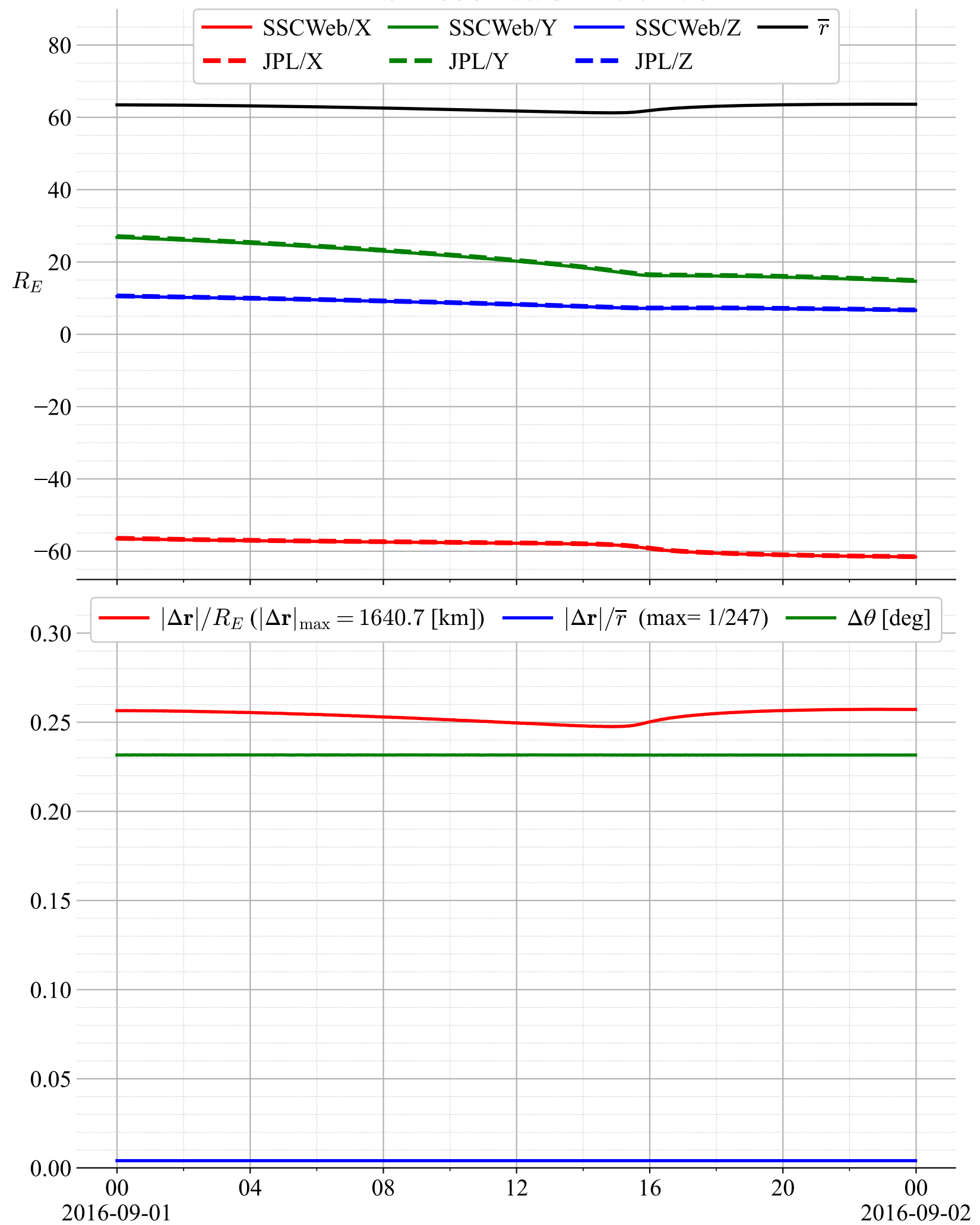
THEMIS-B SSCWeb/GEI vs. JPL/GEI
