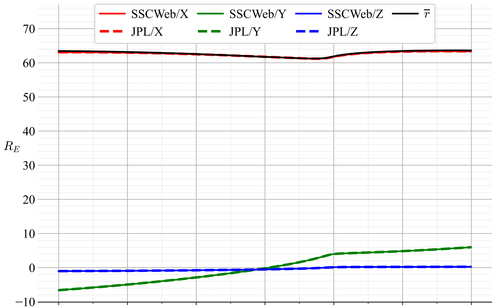
THEMIS-B SSCWeb/GSE vs. JPL/GSE
