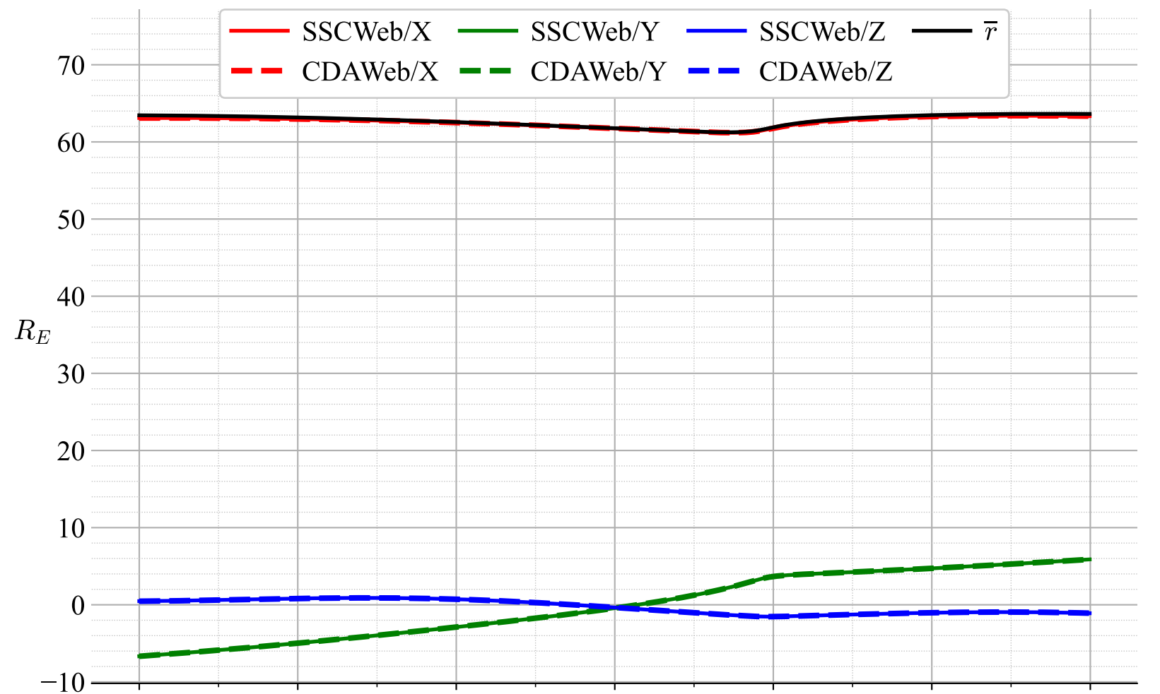
THEMIS-B SSCWeb/GSM vs. CDAWeb/GSM
