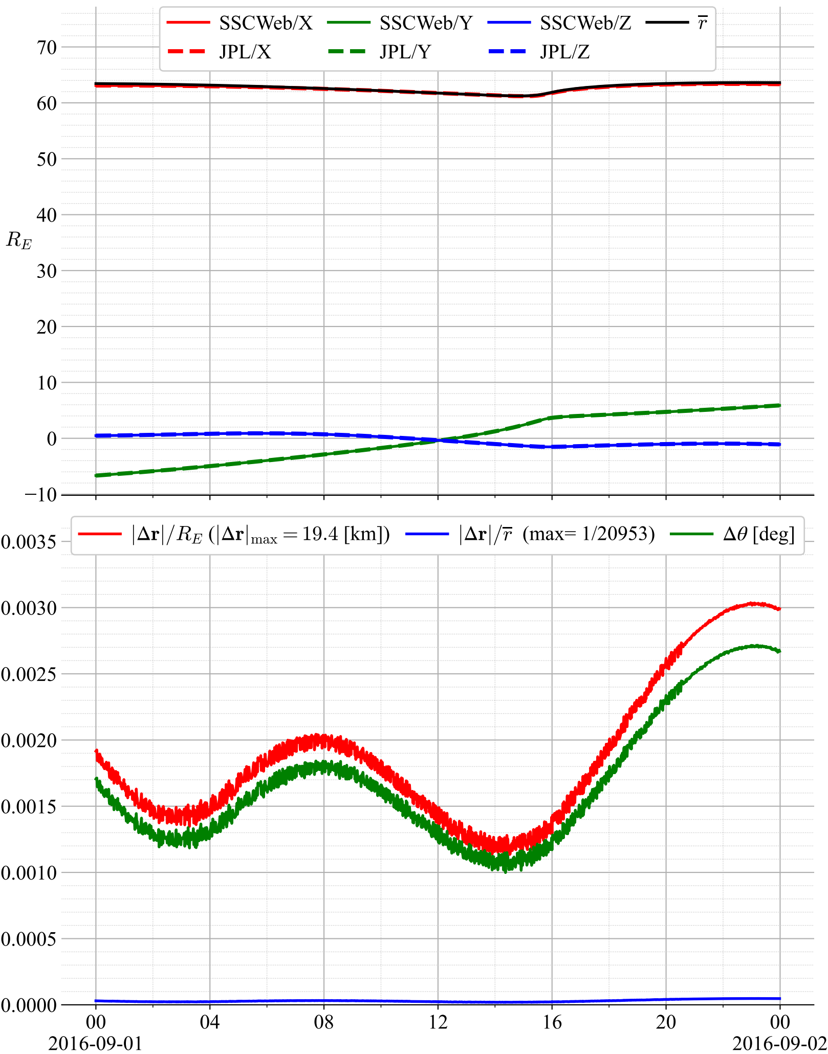
THEMIS-B SSCWeb/GSM vs. JPL/GSM
