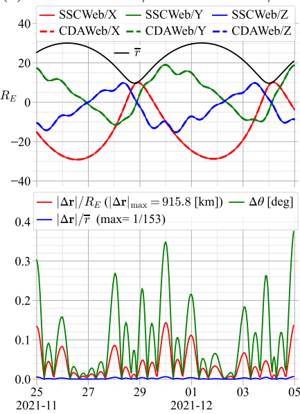
(d) Geotail SSCWeb/GSM vs. CDAWeb/GSM
