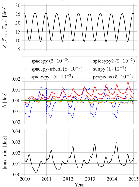
(b) \angle(Z_{\text{GEO}}, Z_{\text{GSM}})
