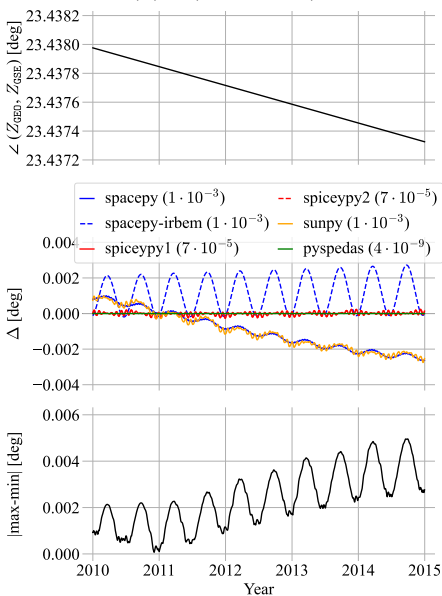
(a) \angle(Z_{\text{GEO}}, Z_{\text{GSE}})
