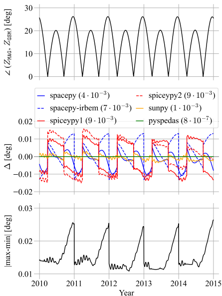
(d) \angle(Z_{\text{MAG}}, Z_{\text{GSM}})
