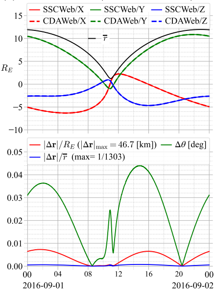
(b) MMS-2 SSCWeb/GSM vs. CDAWeb/GSM
