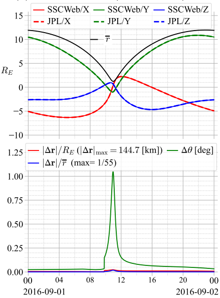
(d) MMS-2 SSCWeb/GSM vs. JPL/GSM
