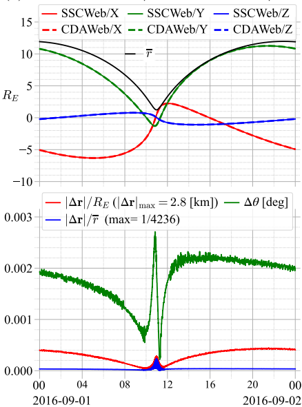
(a) MMS-2 SSCWeb/GSE vs. CDAWeb/GSE
