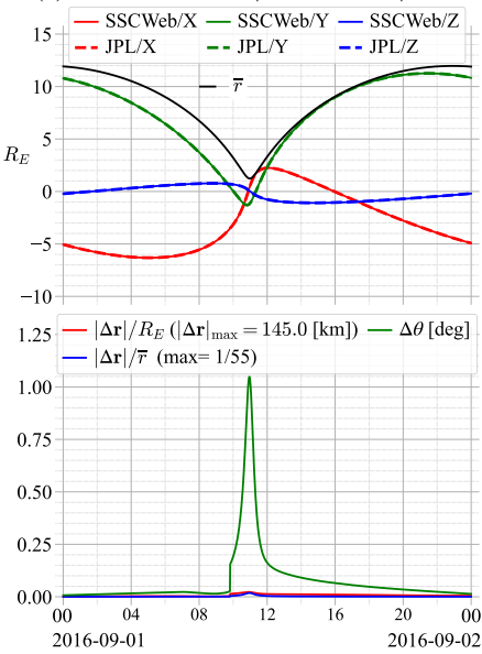
(c) MMS-2 SSCWeb/GSE vs. JPL/GSE
