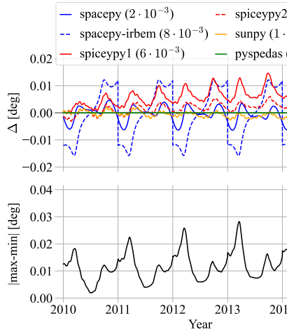
(d) \angle(Z_{\text{MAG}}, Z_{\text{GSM}})
