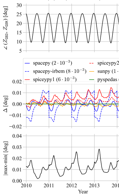
(b) \angle(Z_{\text{GEO}}, Z_{\text{GSM}})
