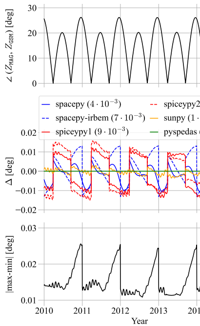
(d) \angle(Z_{\text{MAG}}, Z_{\text{GSM}})
