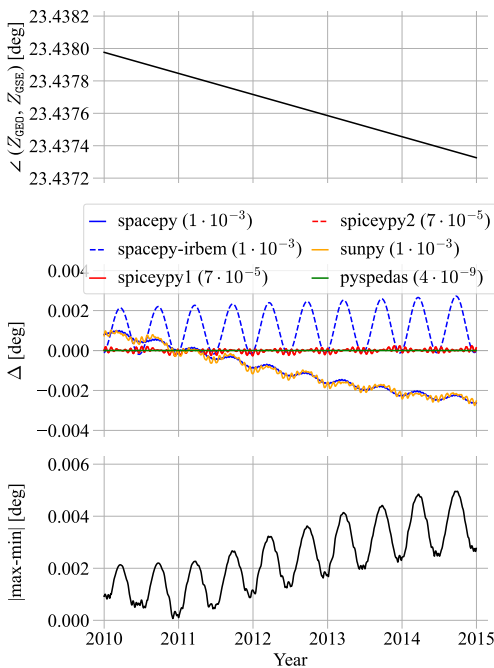
(a) \angle(Z_{\text{GEO}}, Z_{\text{GSE}})
