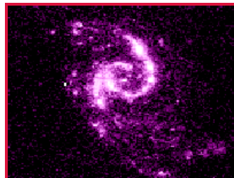
3 Spiral Galaxies
