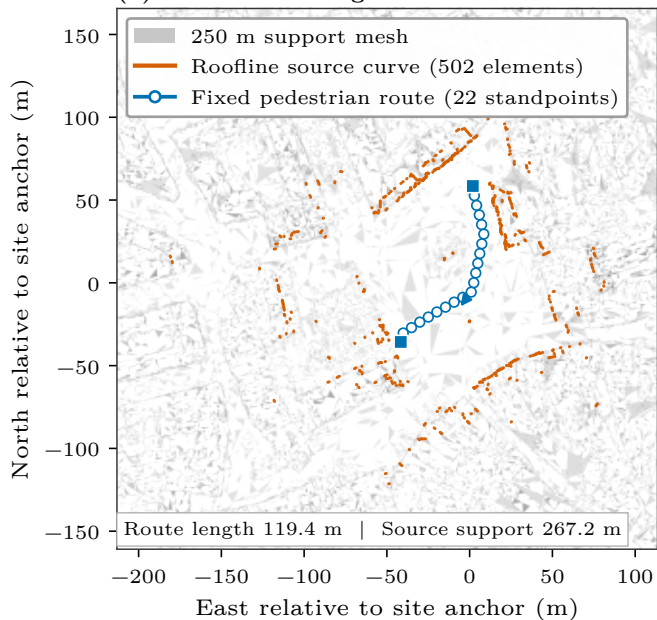
(d) Simulation configuration
