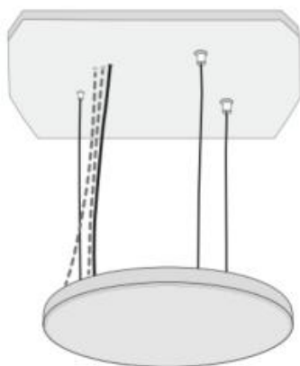
方式3：钢丝绳挂在天花板下
