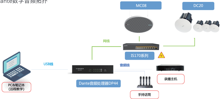
Dante数字音频拓扑
