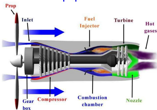
Turbopropulseur
