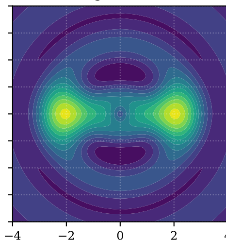
(d) Wave-Ring Emission ( t = 48\tau_0 )
