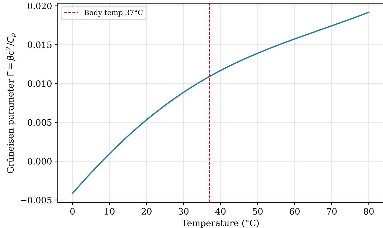
Grüneisen parameter \Gamma vs temperature (water)
