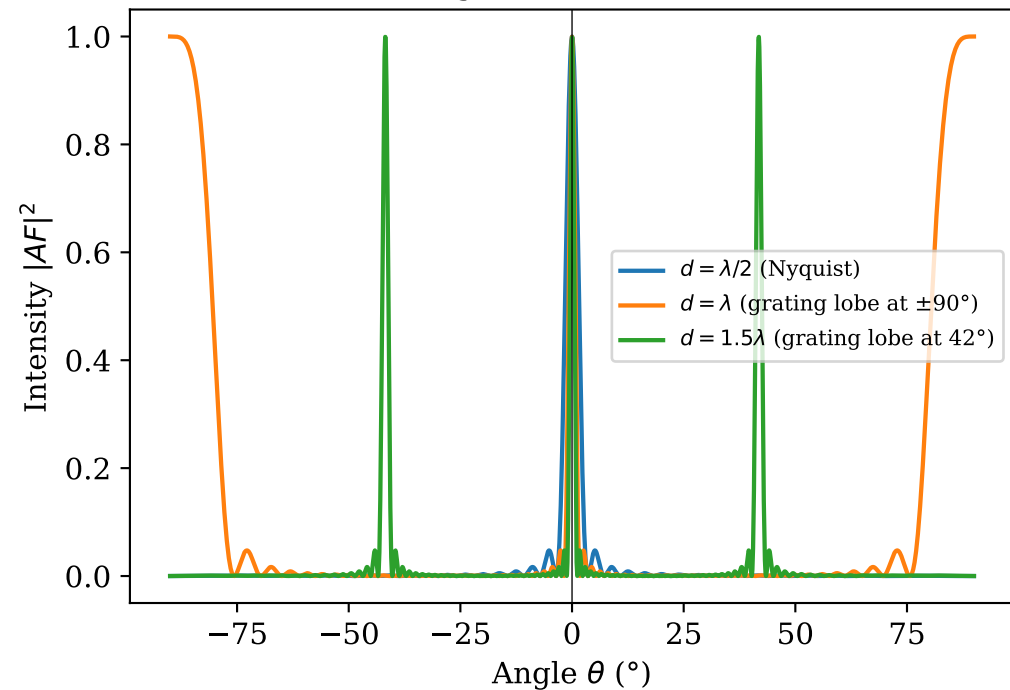
Grating lobes (linear scale)
