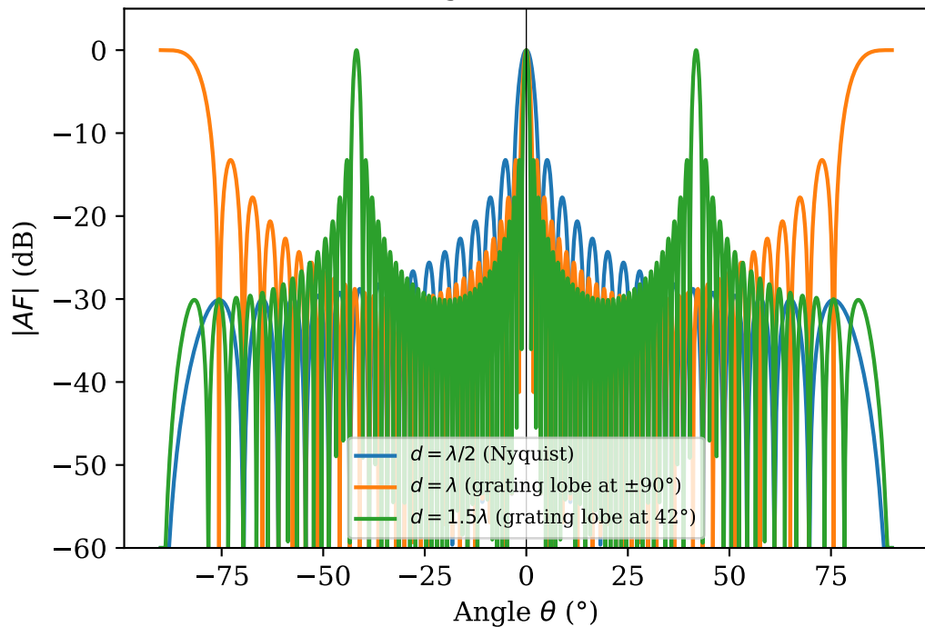
Grating lobes (dB scale)
