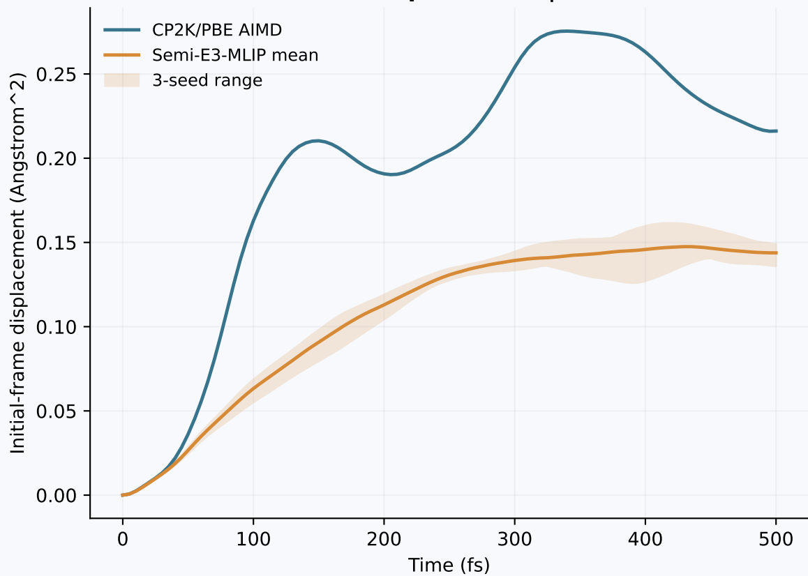
COM-corrected displacement | not diffusion
