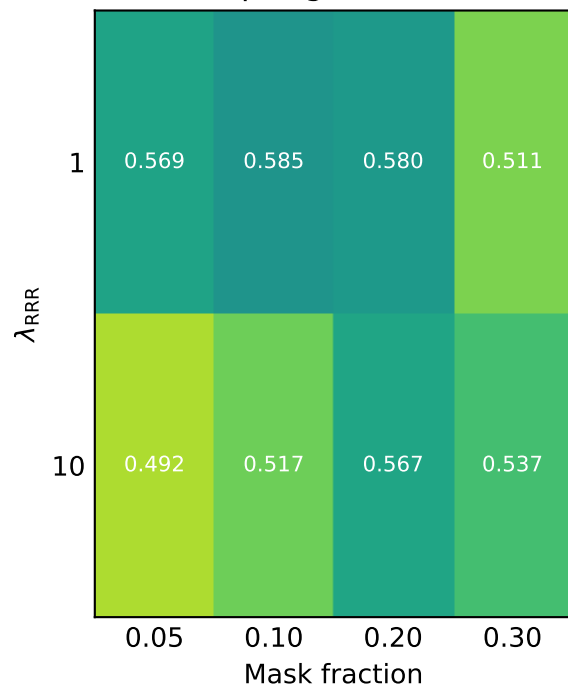
Input gradients
