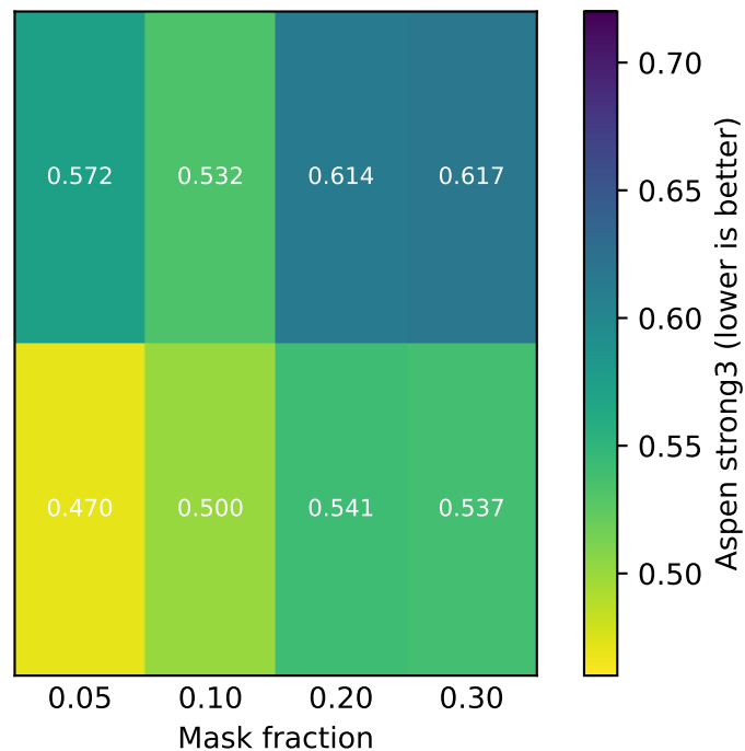
SmoothGrad
