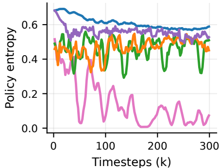
CartPole v1
