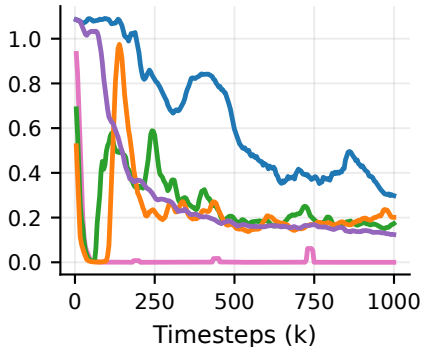
Acrobot v1
