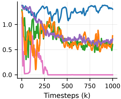
LunarLander v3
