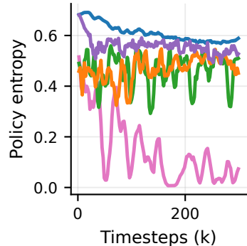
CartPole v1
