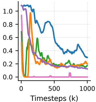
Acrobot v1
