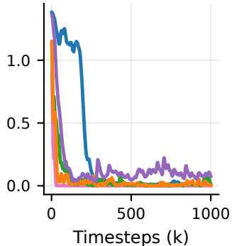
FrozenLake v1
