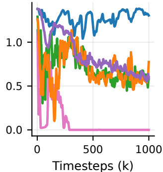
LunarLander v3
