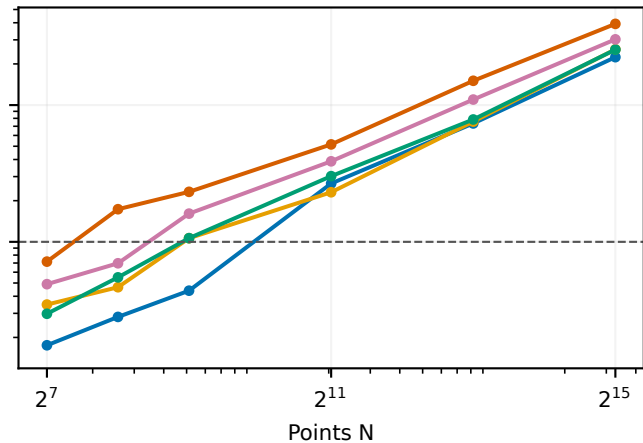
Halton inputs
