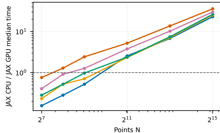
Sobol inputs
