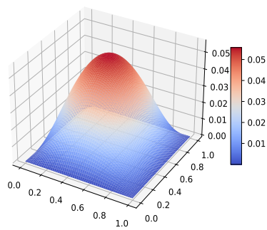
図 5.2 \epsilon = 0.06 の \hat{v}
