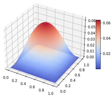
図 5.6 \epsilon = 0.047 の \hat{v}
