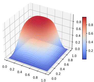
図 5.3 \epsilon = 0.05 の \hat{u}
