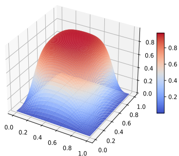
図 5.5 \epsilon = 0.047 の \hat{u}
