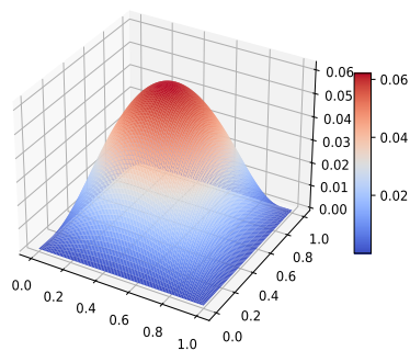
図 5.4 \epsilon = 0.05 の \hat{v}
