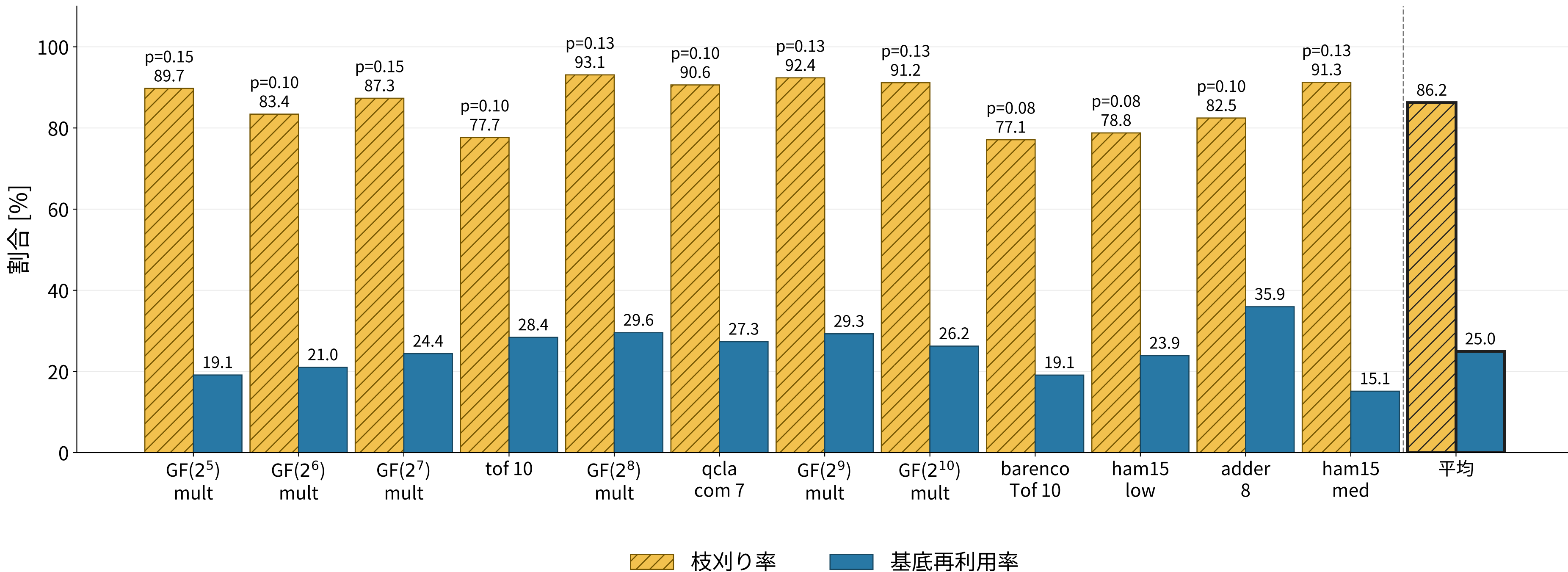
最速設定における枝刈り率と基底再利用率
