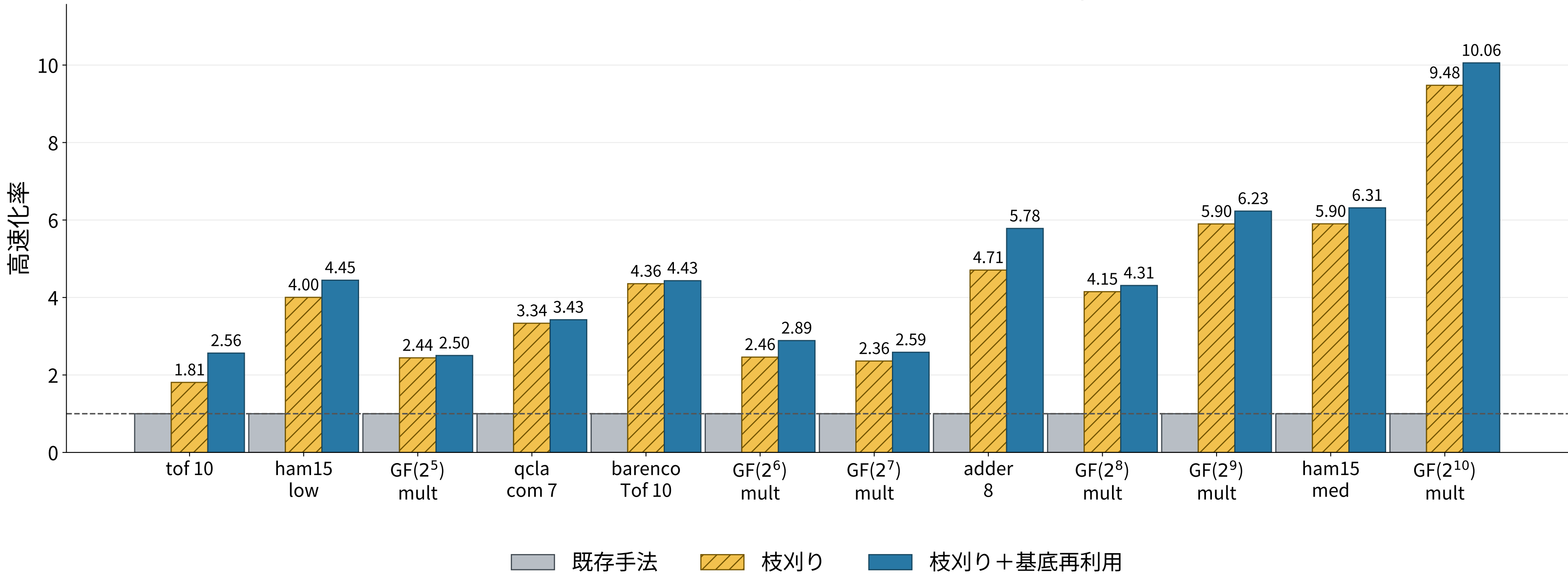
自前ビット並列実装を基準とした高速化率
