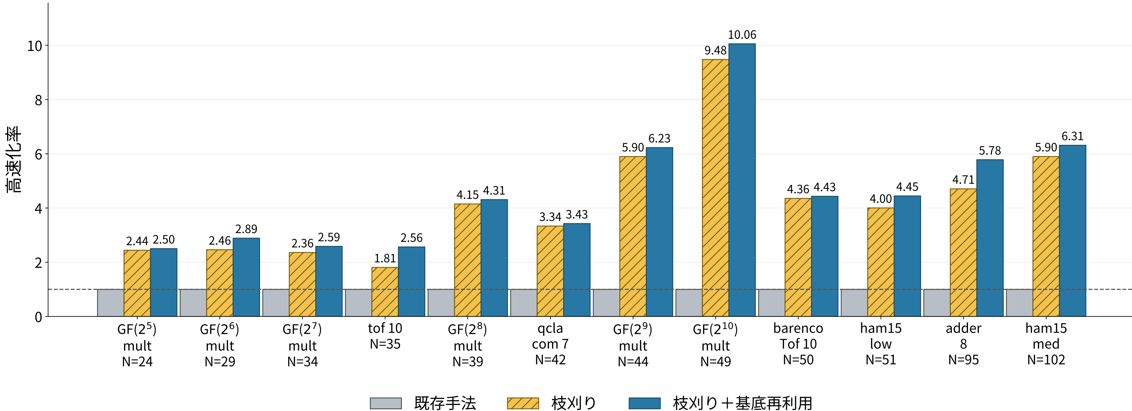
TODD総量子ビット数順の高速化率
