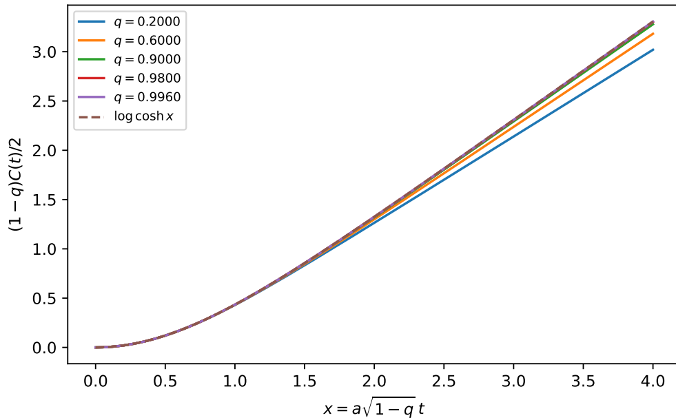
図 1 同じ無次元時間で比較した Krylov complexity。破線は fit を行わずに式 (5.1) から得た曲線である。
