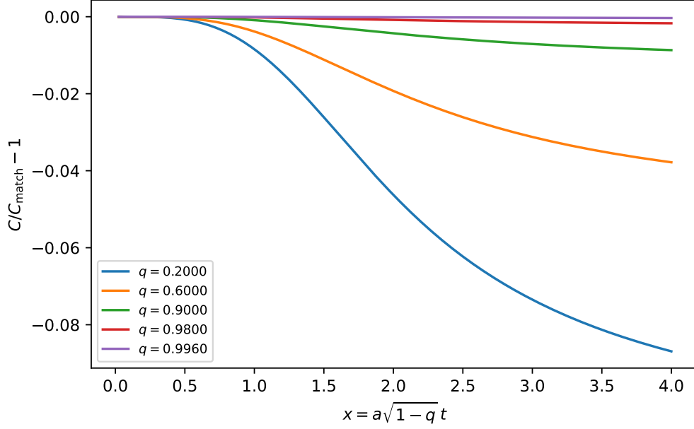
図2 式 (5.1) からの相対偏差。 q \rightarrow 1 で偏差が小さくなる。この図だけで全時間一様な収束を証明したことにはならない。
