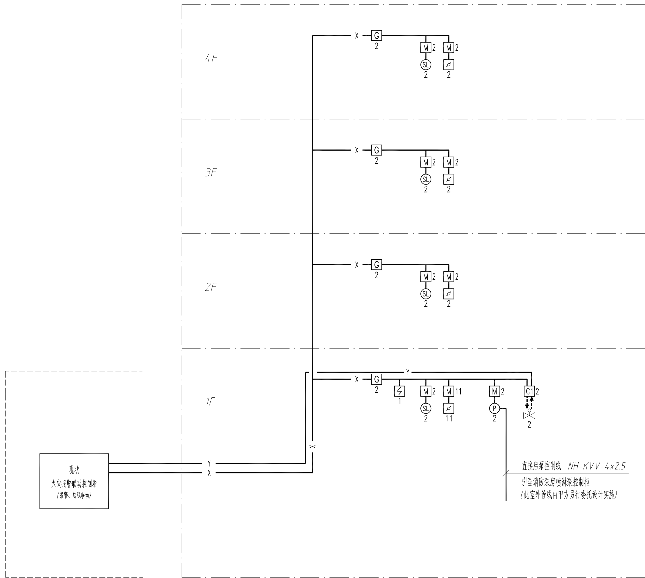
火灾自动报警及联动系统图
