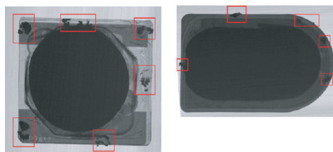
検査結果画像:部分印刷フィルムおよび全面印刷フィルムにおけるシール部コンタミの検出例
