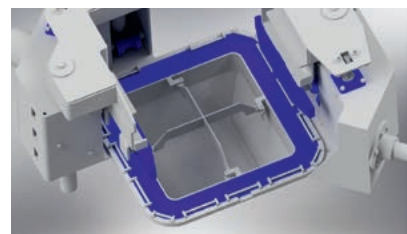
蓋内側のミキシングクロス / トロリータンブラー
