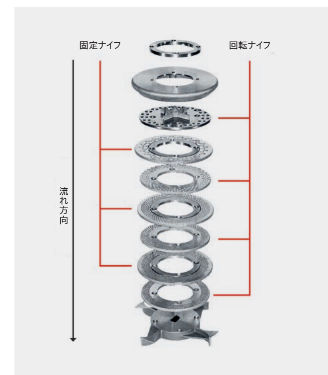
コンティカッター 250 ホールプレート セット例
